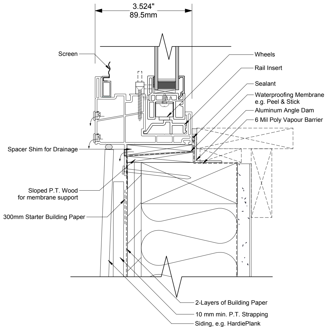
1 Slider Sill Detail Scale: 1:2
